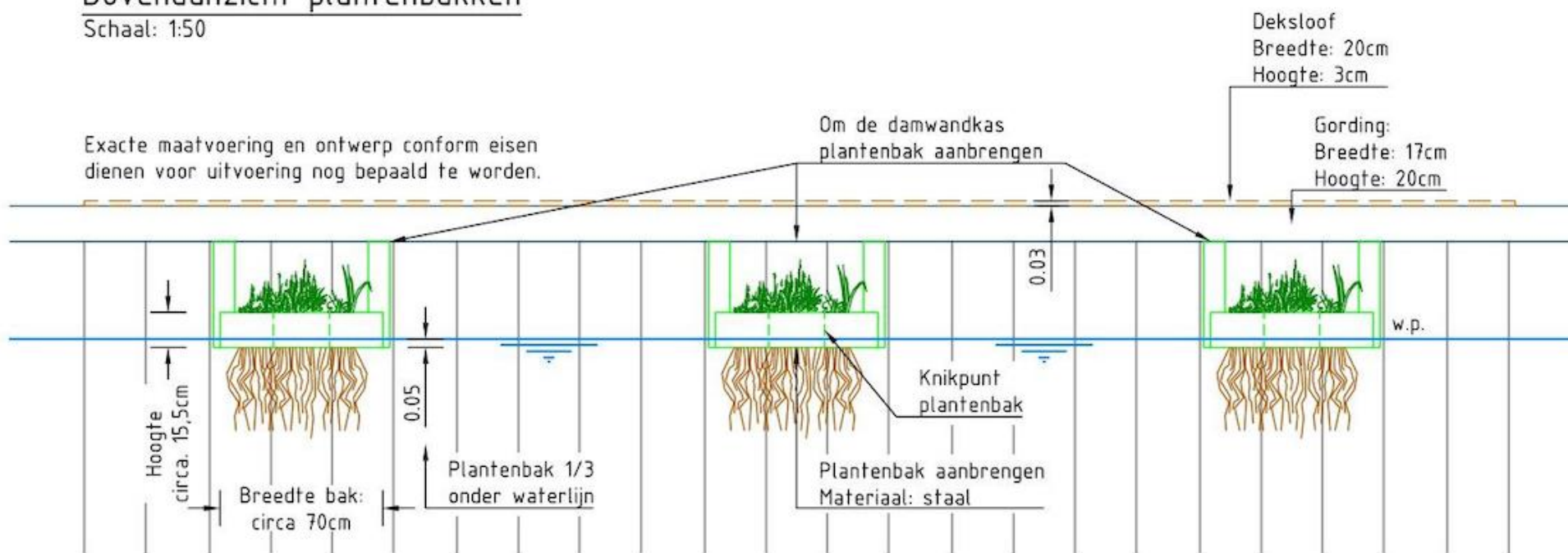
Vooraanzicht plantenbakken Schaal: 1:50
