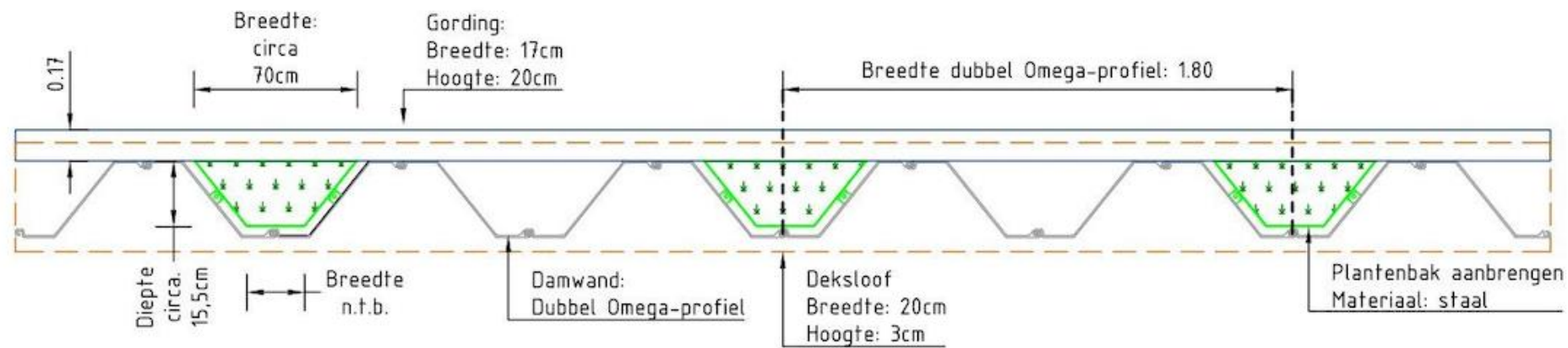
Bovenaanzicht plantenbakken Schaal: 1:50
