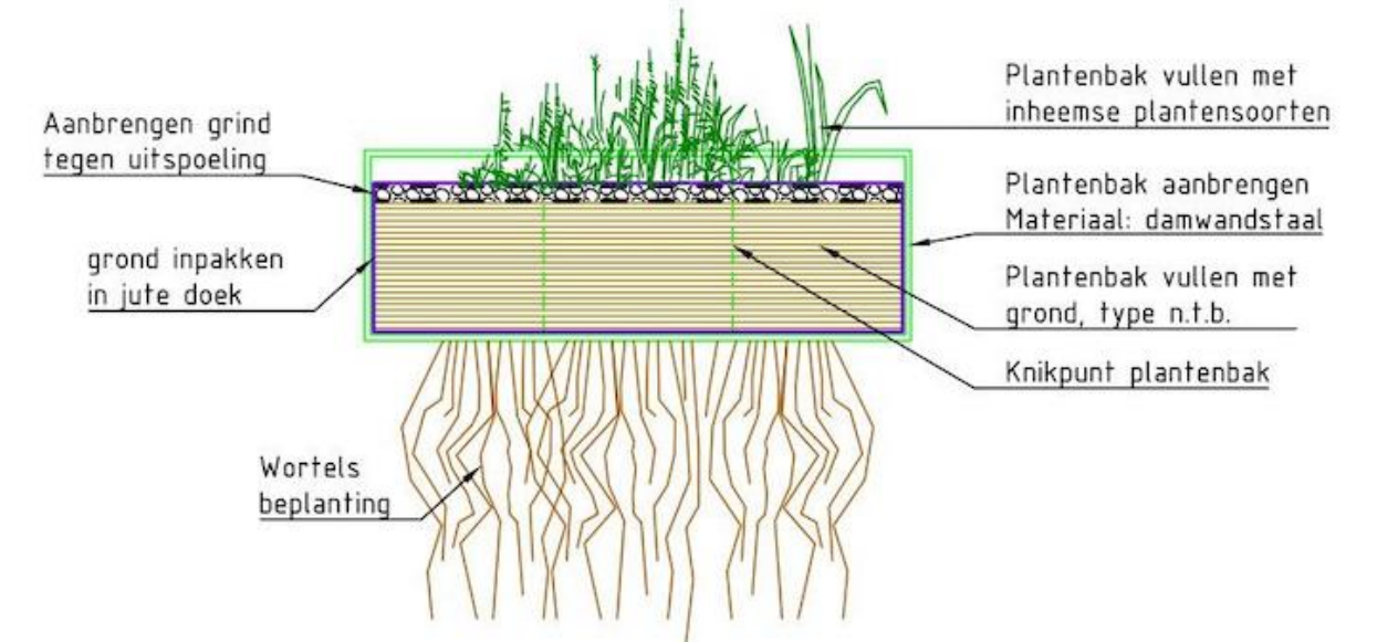
Principe detail plantenbak Schaal: 1:20
